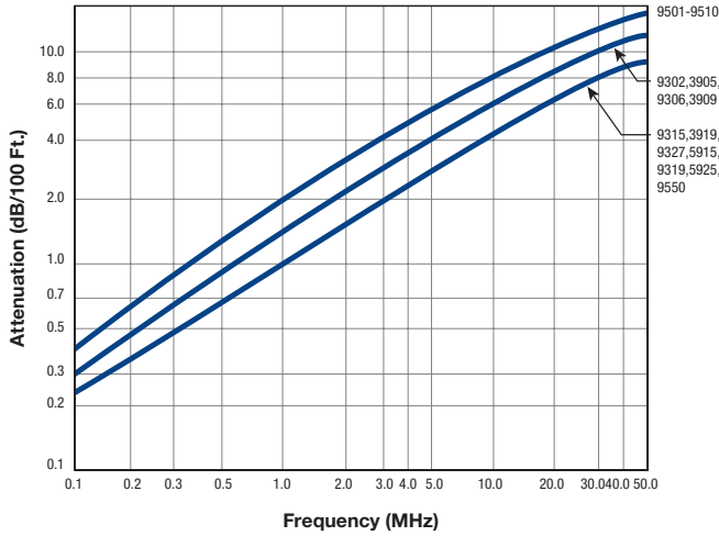
Attenuation
